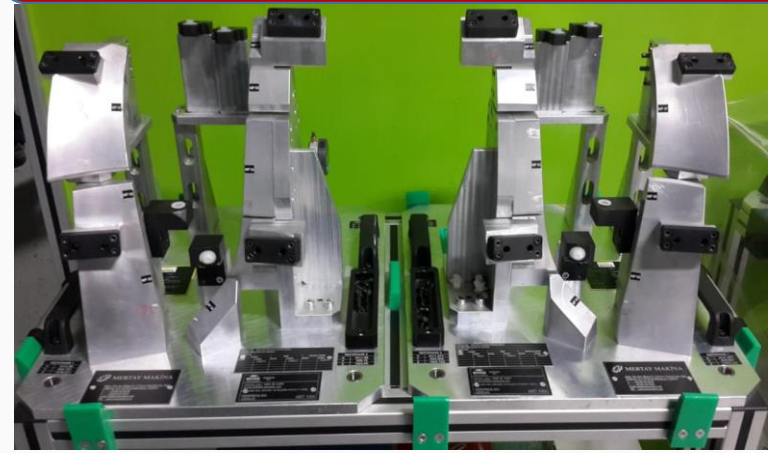
1D ÖLÇÜM CİHAZI
